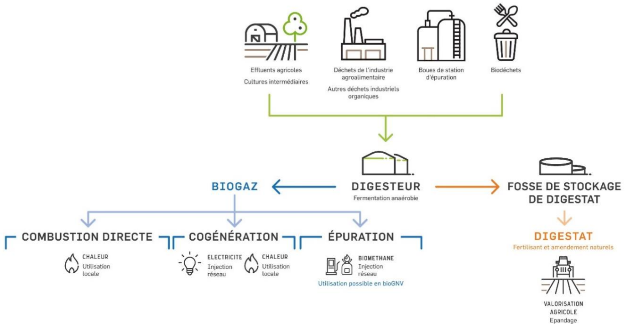
Figure 1 : Le processus de méthanisation - Métha'Synergie
